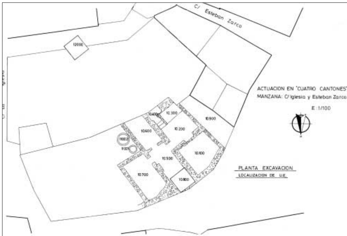
Figura 3. Solar 1, Planta del yacimiento y delimitación de U.U.E.E.
