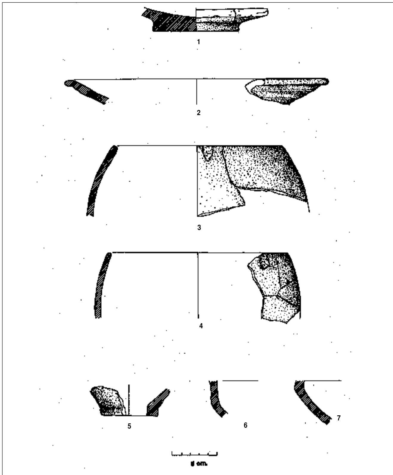
Fig. 4. Fondo plano de plato de cerámica gris (fig. 4.1), fragmento de plato de borde vuelto de cerámica gris (fig. 4.2), ollas u orzas con mamelones de aprehensión verticales pendientes del borde (ff. 4.3 y 4.4), fondo plano de pequeña olla u orza (fig. 4.5), fragmento de cazuela carenada de cerámica gris (fig. 4.6) y fragmento de escudilla carenada de cerámica gris (fig. 4.7).
