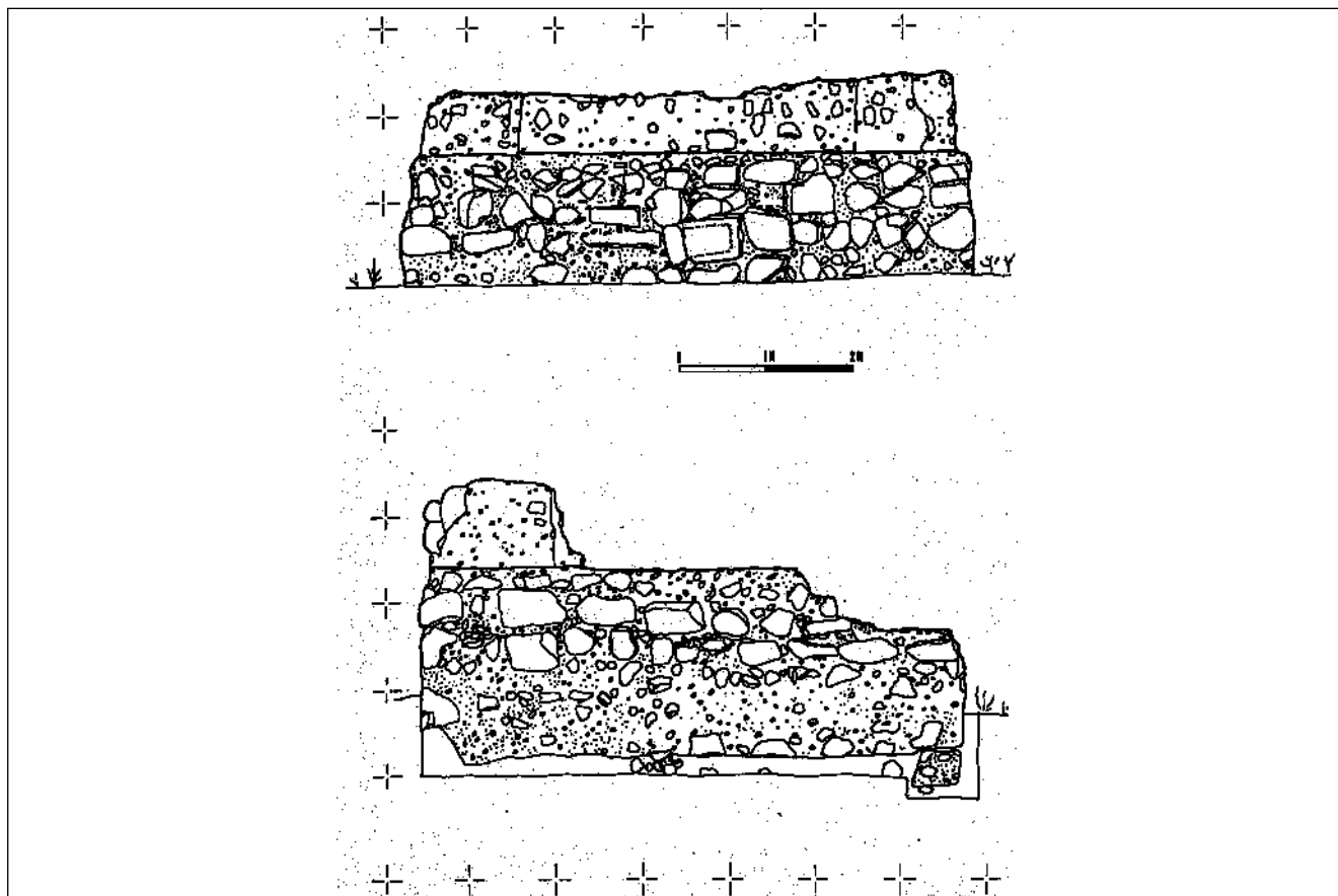
Fig. 6. Alzados y cimentación de las caras Sureste y Noroeste de la Torre de Sancho Manuel.
