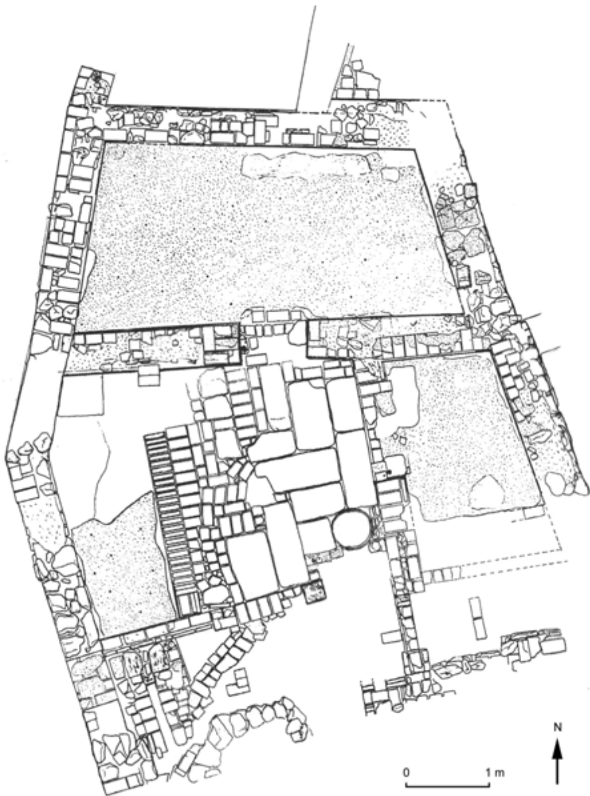
Figura 6.- Planta arqueológica de la casa A en la fase III.
