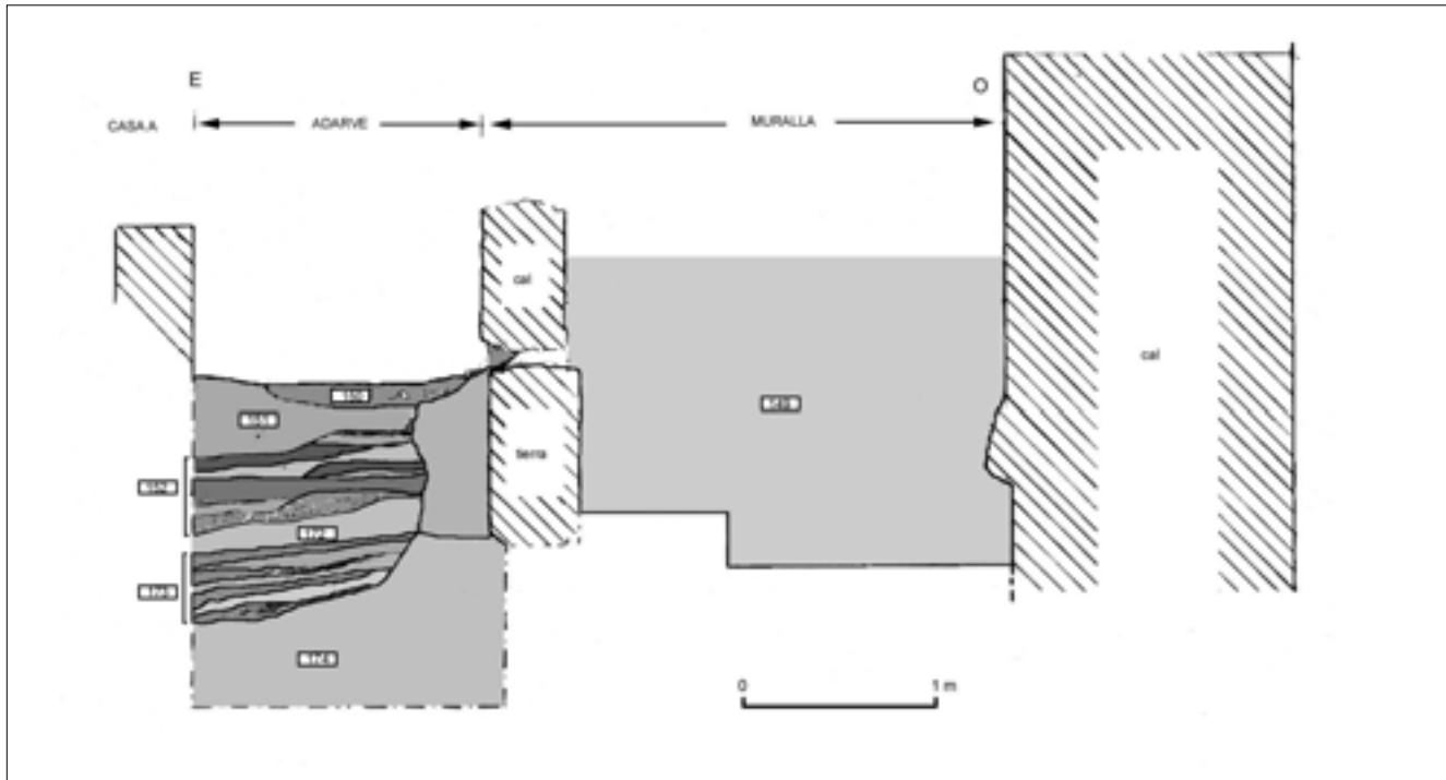
Figura 4.- Sección transversal del adarve y la muralla.
