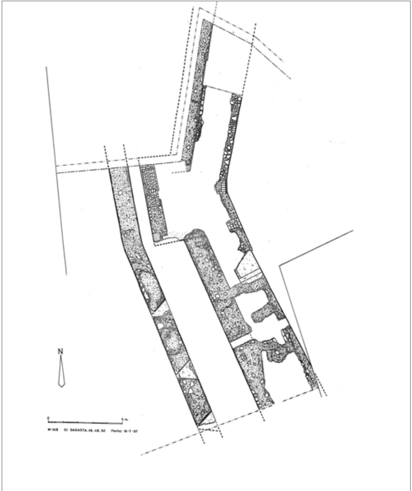
Figura 3.- Planta arqueológica de las construcciones defensivas.
