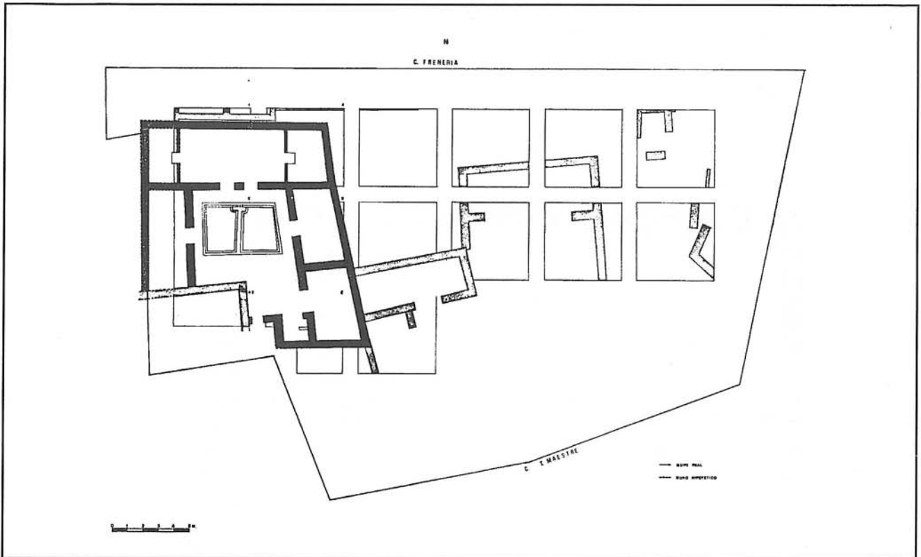
Fig. 2.- Primer momento constructivo.
