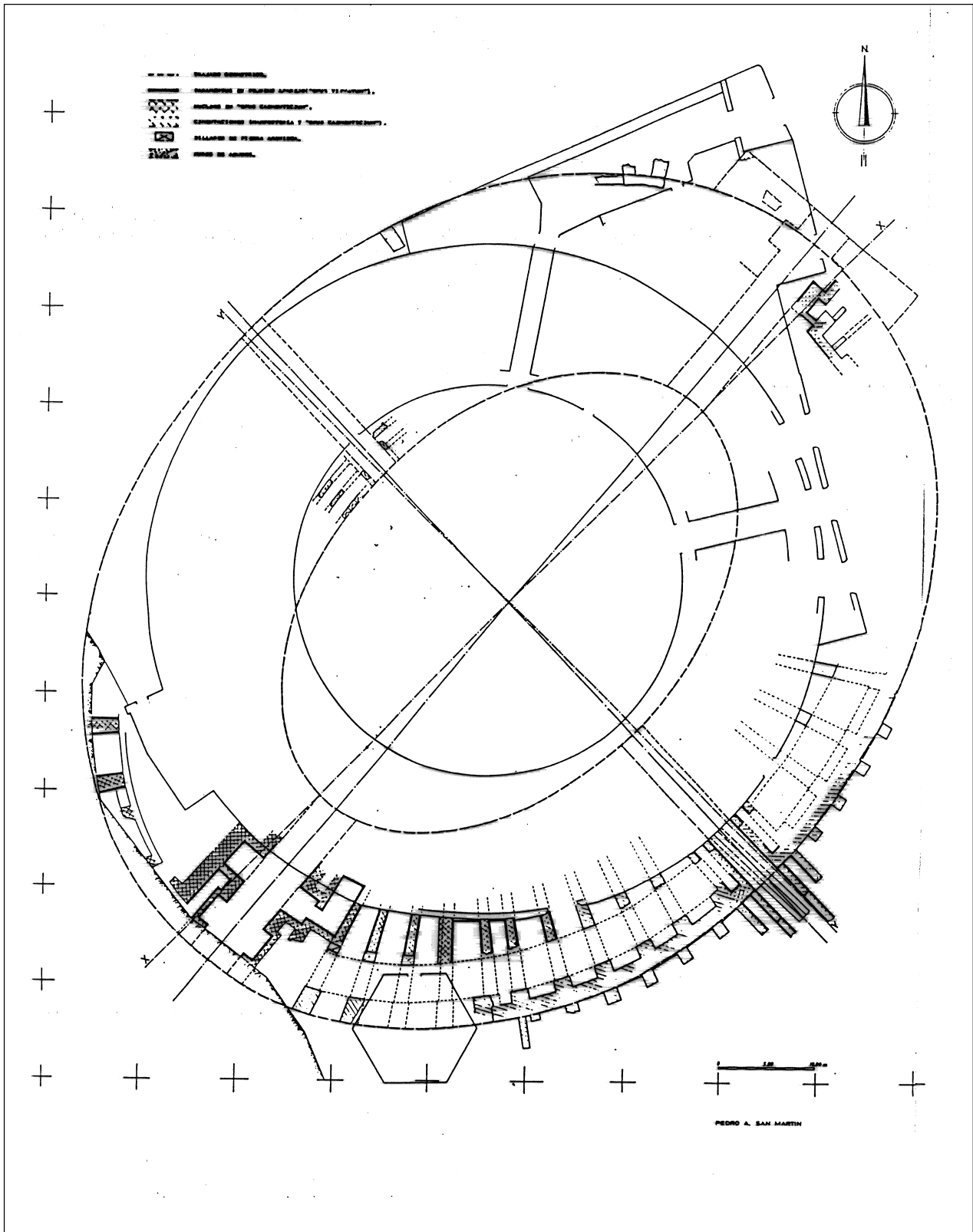
Lámina 8. Planta del anfiteatro romano tras la intervención de 1991/92.
